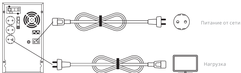
Рис. 3.2.2. Схема подсоединения входа/выхода напольного ИБП 3000 ВА*
