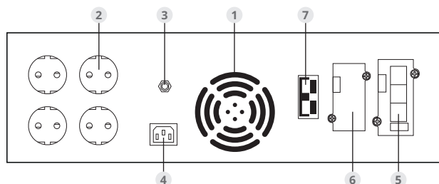
Рис. 2.3.2. Задняя панель ИБП в стойку (ЮНИОР ПРО РТ) 1500 – 3000 ВА 3U
