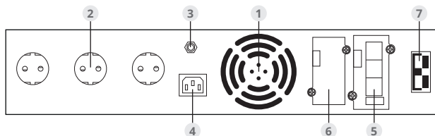
Рис. 2.3.2. Задняя панель ИБП в стойку (ЮНИОР ПРО РТ) 2000 ВА 2U
